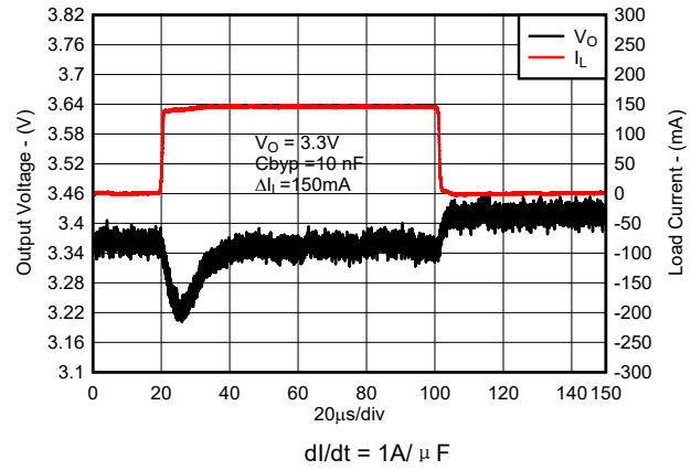
图 7-11. Load Transient (New Chip)
