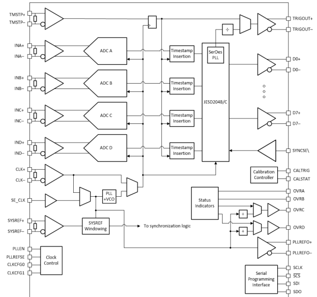
四通道器件方框图
