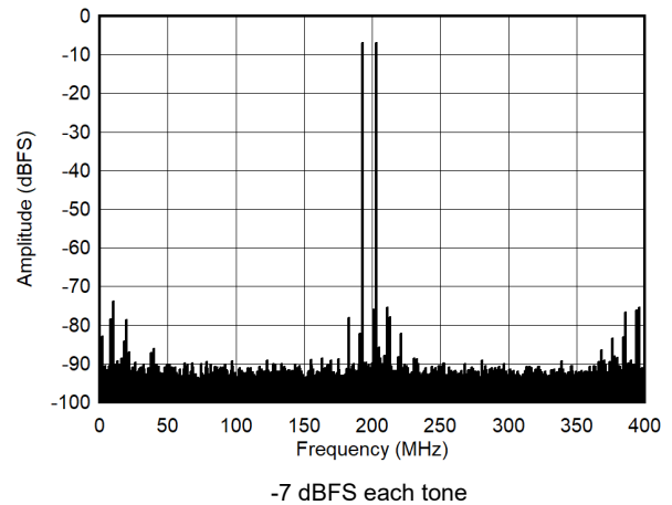
图 7-52. Single Tone FFT at 998 MHz
