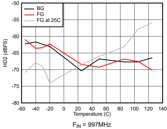
图 7-37. HD2 vs Temperature
