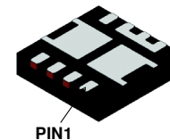
PIN1 WQFN12 3.3X3.3, 0.65P CASE 510CJ
