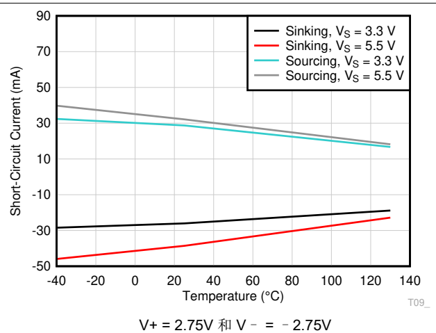
图 6-20. 短路电流与温度间的关系
