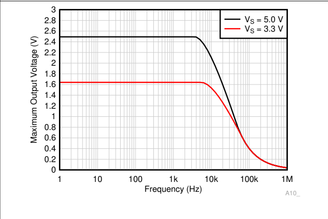
图 6-44. 最大输出电压与频率间的关系
