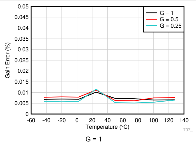
图 6-18. 增益误差与温度间的关系
