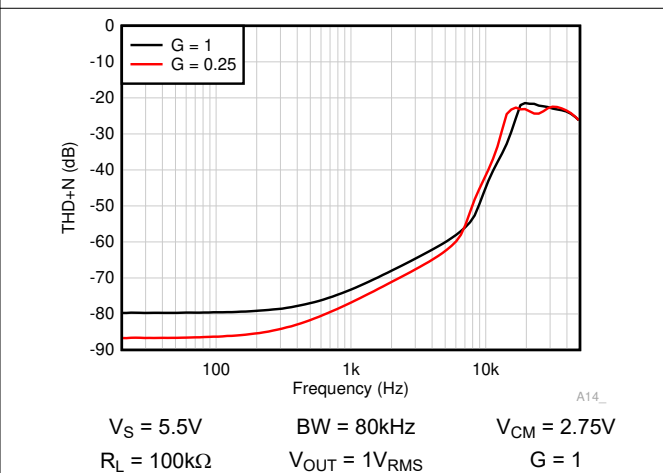
图 6-46. THD + N 与频率间的关系
