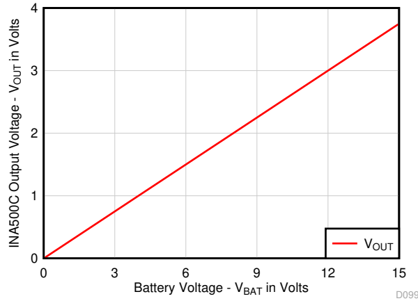
图 8-3. 电池输入电压与 INA500C 输出电压的关系
