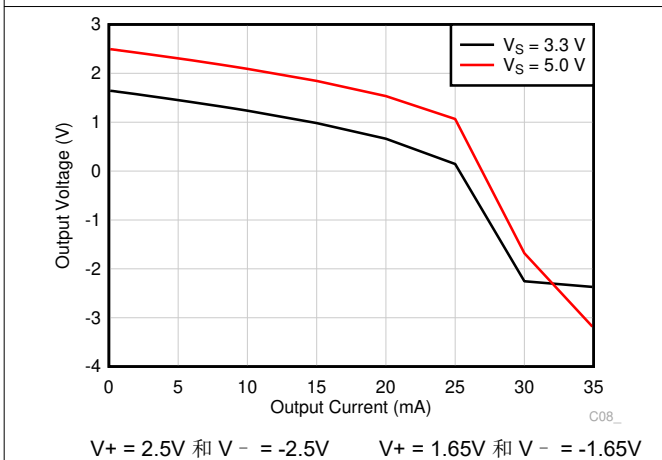
图 6-33. 输出电压与输出电流 (拉电流) 间的关系
