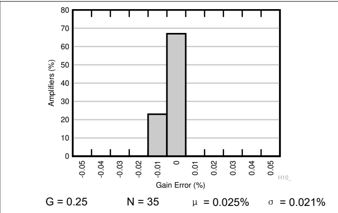
图 6-12. 增益误差的典型分布
