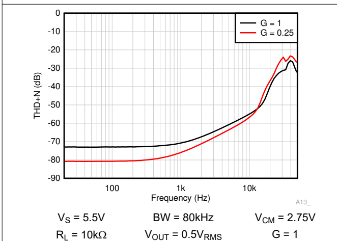
图 6-45. THD + N 与频率间的关系
