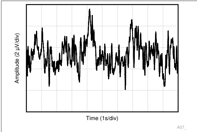
图 6-41. 以输出为基准的 0.1Hz 至 10Hz 时域电压噪声
