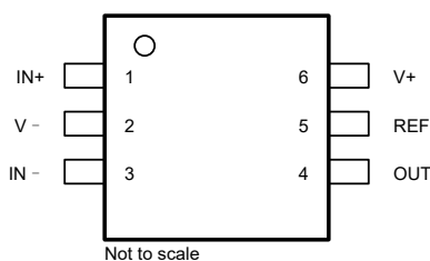
图 5-1. INA500 DCK 封装，6 引脚 SC70 (顶视图)
