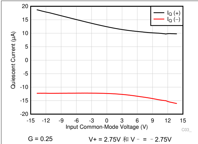
图 6-29. 静态电流与输入共模电压间的关系
