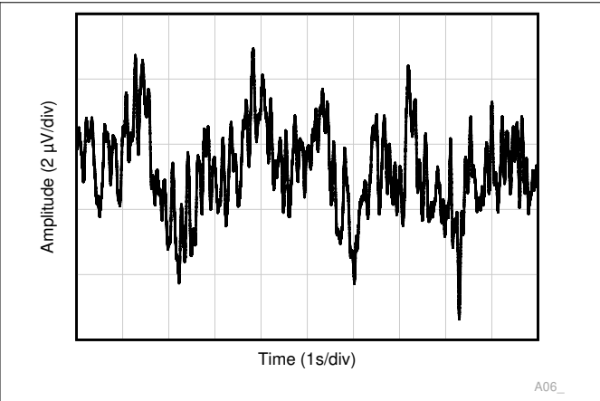
图 6-42. 以输出为基准的 0.1Hz 至 10Hz 时域电压噪声
