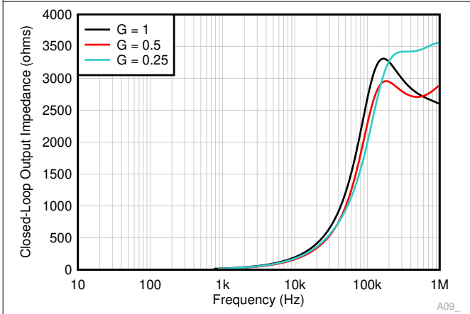
图 6-43. 闭环输出阻抗与频率间的关系
